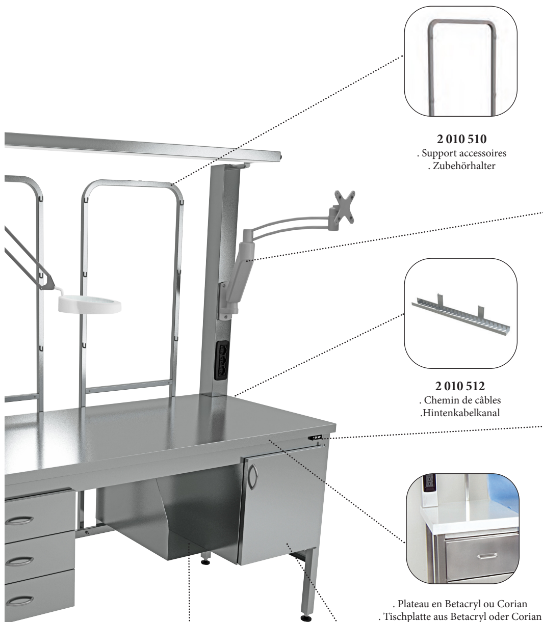
2 010 540 · Support écran · Bildschirmhalter
